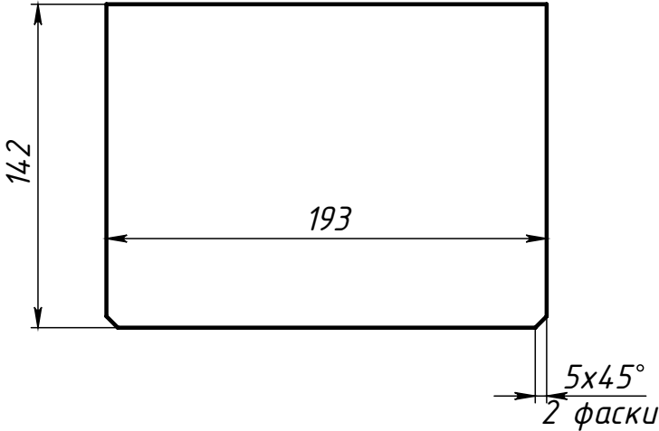
Поз.2 (Ребро)
